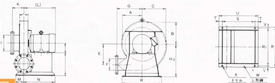
PFO型寸法表
